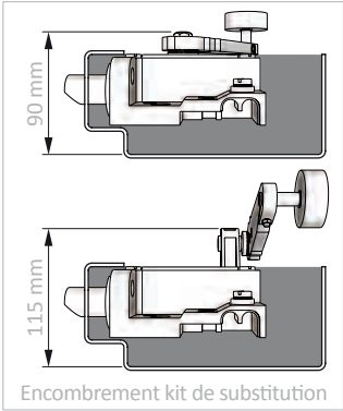
Encombrement kit de substitution
