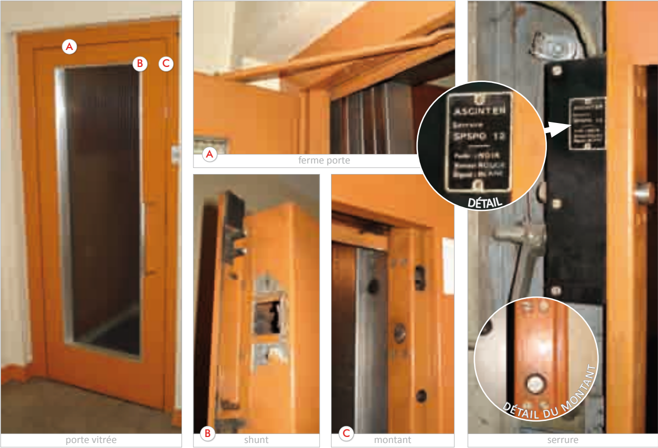
ex : serrure droite sur porte OTIS
