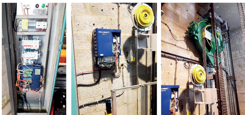
KONE MONOSPACE - 1000 kg - 1.00 m/s
